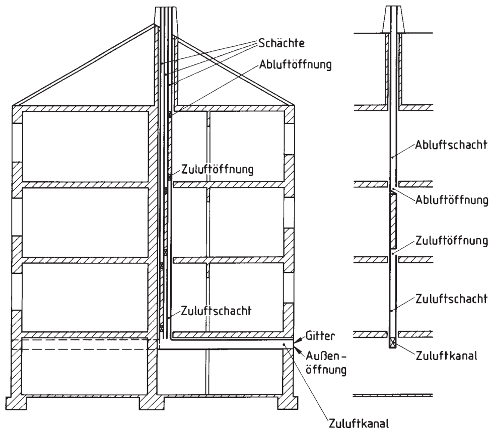
Bild 1. Einzelschachtanlage (Beispiel)
